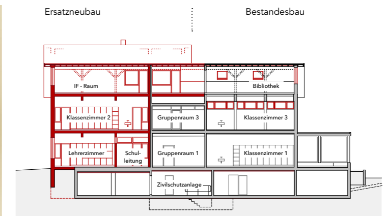
Längsschnitt A-A
